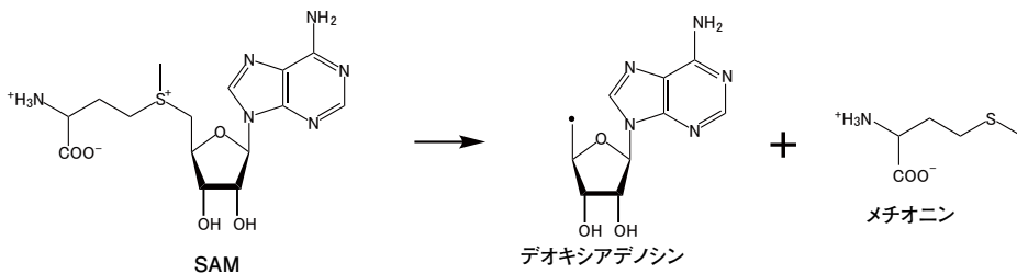
SAMが開裂して、デオキシアデノシンとメチオニンになる反応
