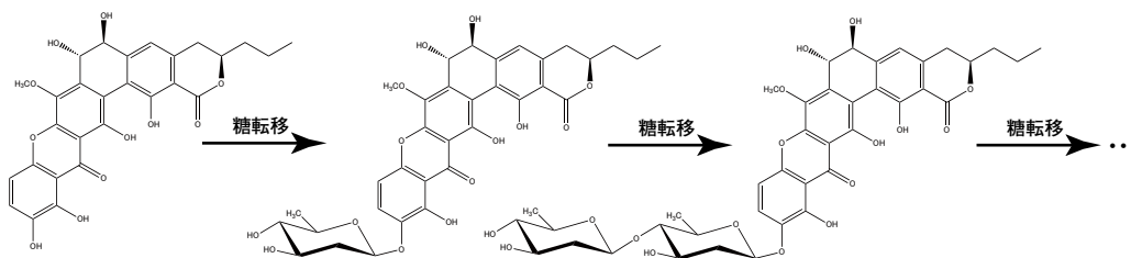
図5 糖転移反応による基質の構造変化
