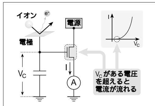
図4 イオンカウンター回路図
